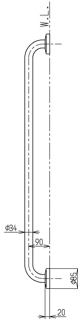
取付座詳細(1:2)
