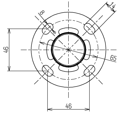
取付座詳細(1:2)
